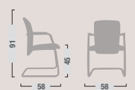
KL 27 Sedia fissa con braccioli. Fixed armchair.
