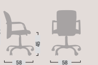
KL 24 Sedia girevole con braccioli. Swivel armchair.
